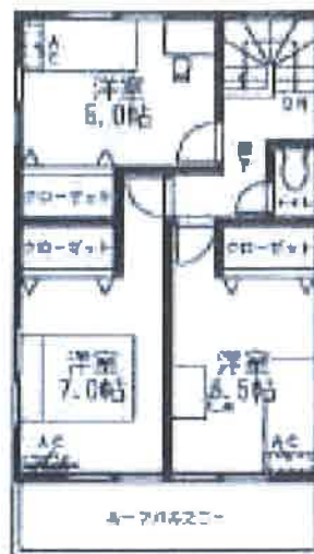
2階平面図：44.72㎡
