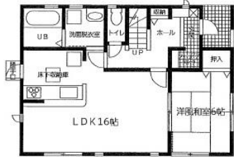
1階平面図:55.48㎡
